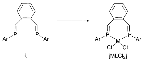
Scheme 1 Ar = C 6 H 2 Bu t 3-2,4,6 ; M = Pd, Pt
